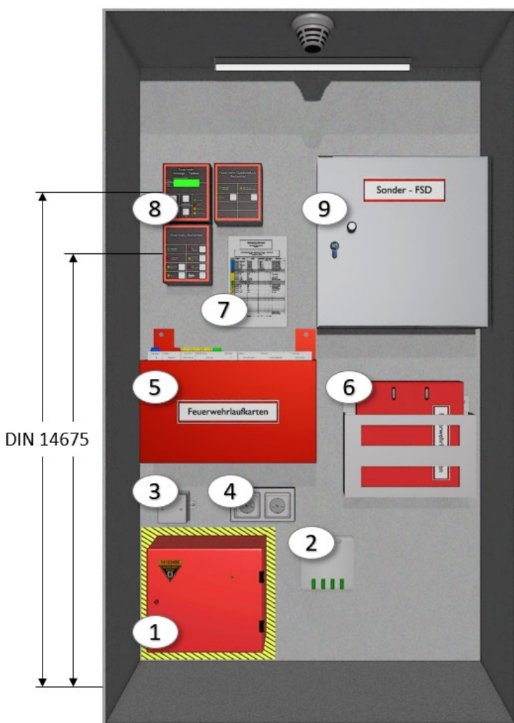
Schematische Darstellung der BMZ
