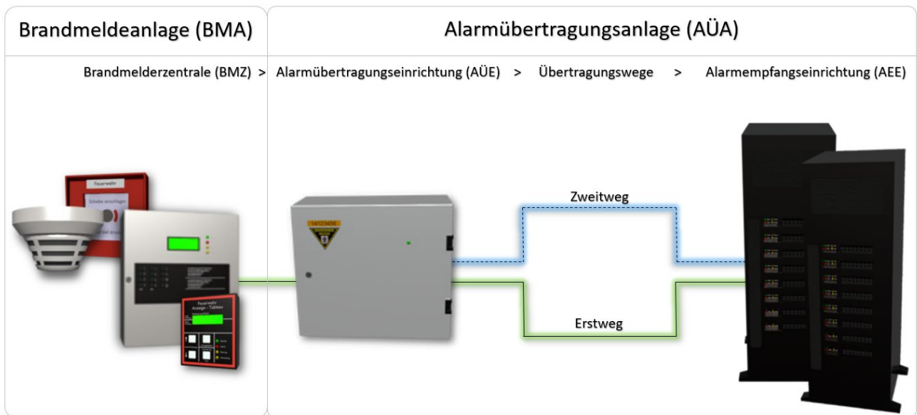
Abbildung 4-1: Schematische Darstellung AÜA
