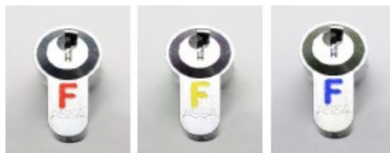
Abbildung 6-1: Profilhalbzylinder der Feuerwehrschießung München
