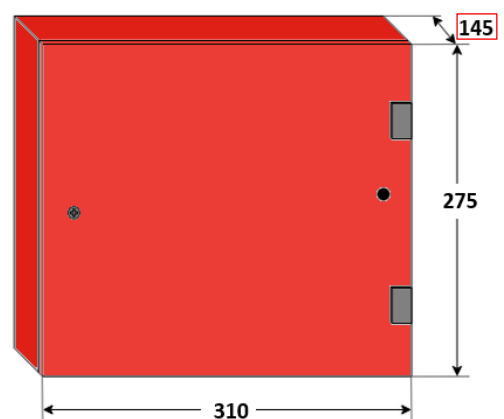
Abmessungen der Alarmübertragungseinrichtung (AÜE), Maße in Millimeter
